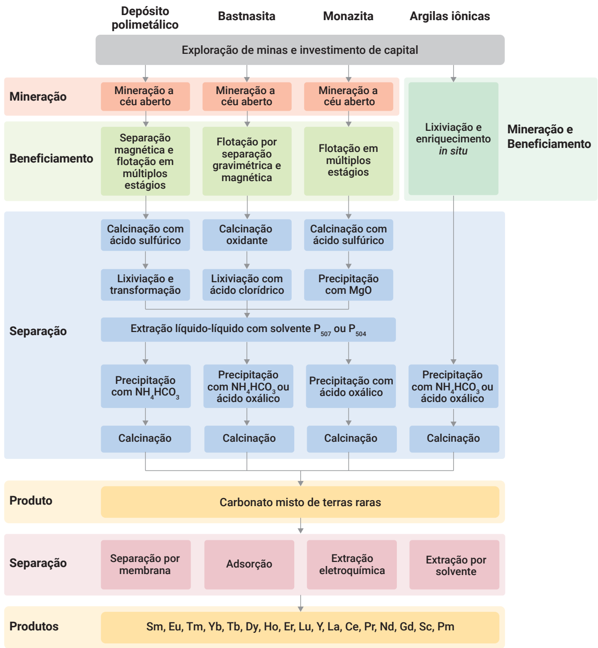
FIGURA 2 Rotas tecnológicas de processamento para ETR
